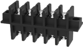
DG30-A Pitch: 13mm
